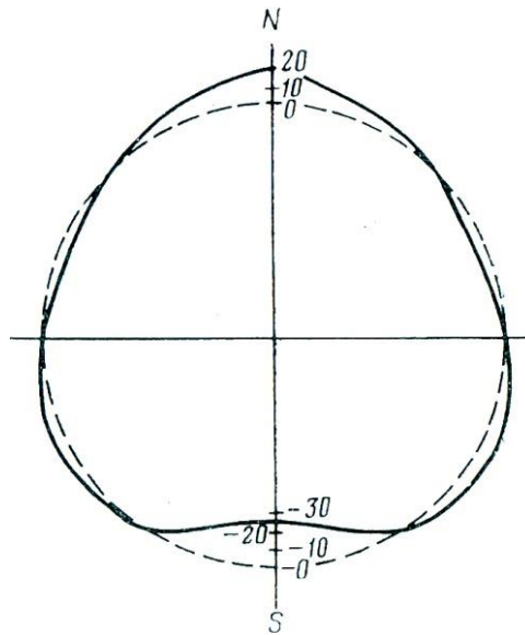
Рис. 20. Меридиональное сечение Земли (расчёт по данным Д.Г. Кинг-Хили) [5, с. 114]
