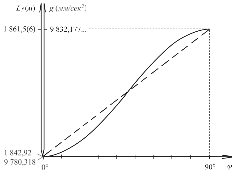
Рис. 21. Графики изменения длины угловой минуты меридиана L_1' и ускорения свободного падения g от географической широты \varphi [12, с. 45-46]
